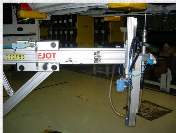
Sistema móvel, semi-automático de aperto controlado
